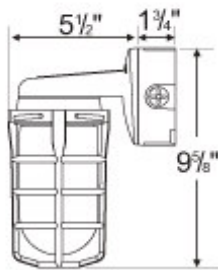
VP101-W (Wall Mount)
